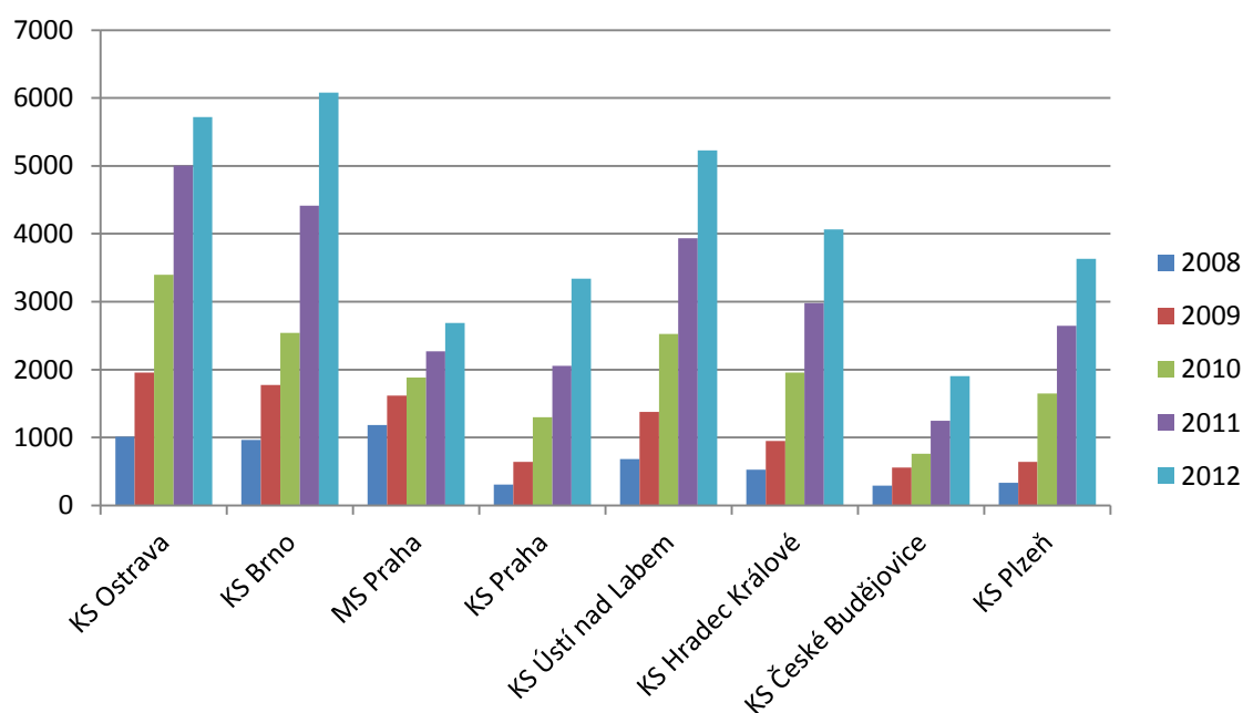
Graf 1 Počty insolvenčních návrhů u jednotlivých insolvenčních soudů
