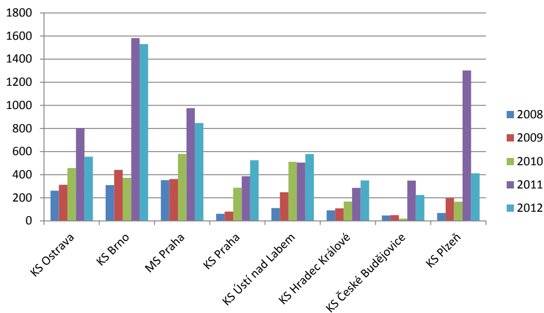
Graf 4 Počet odmítnutých insolvenčních návrhů
