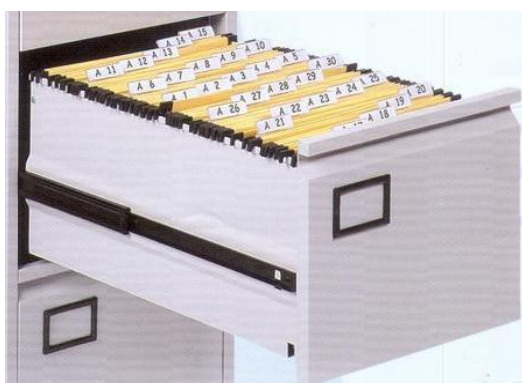
Obrázek 3 - Databáze 5
