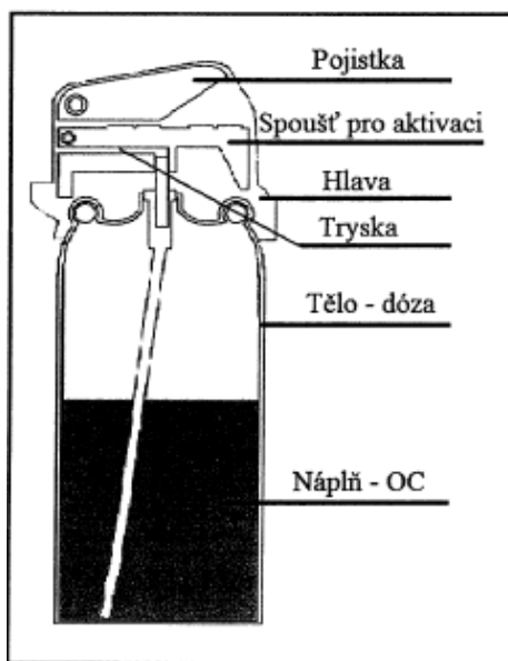
Obrázek 1: Jednotlivé komponenty obranného spreje [32]
