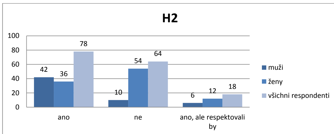
Graf 12: Hypotéza 2
