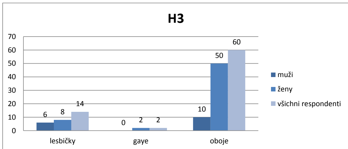
Graf 13: Hypotéza 3
