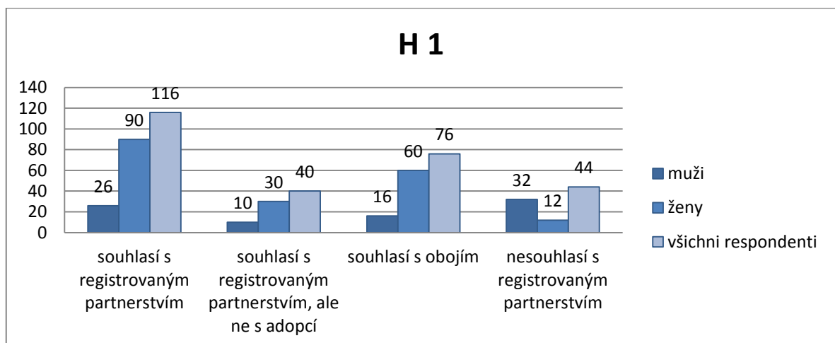
Graf 11: Hypotéza 1
