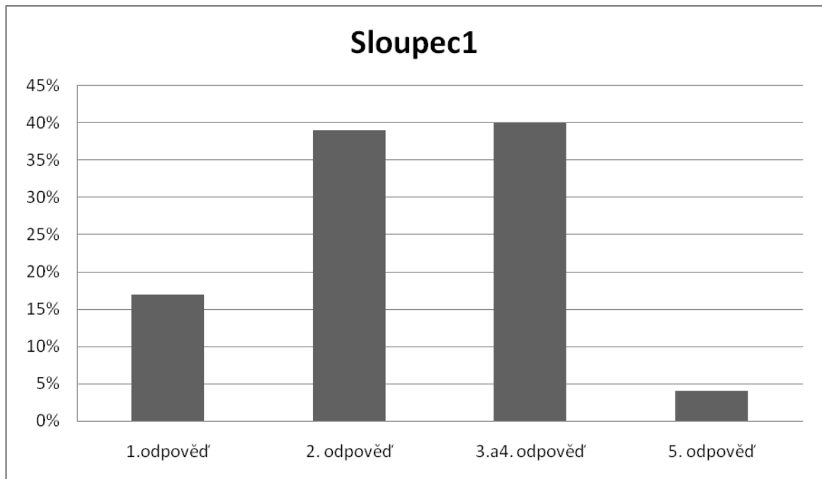
Graf Diskriminace
