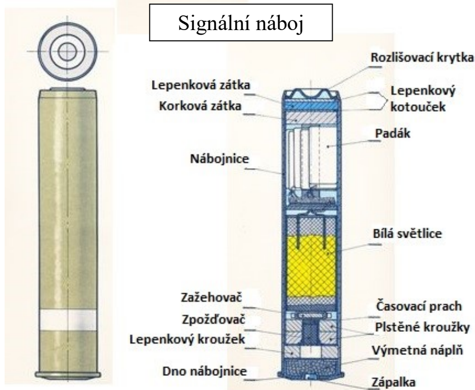
Obr. 4. Signální náboj 26,5mm s popisem [32]
