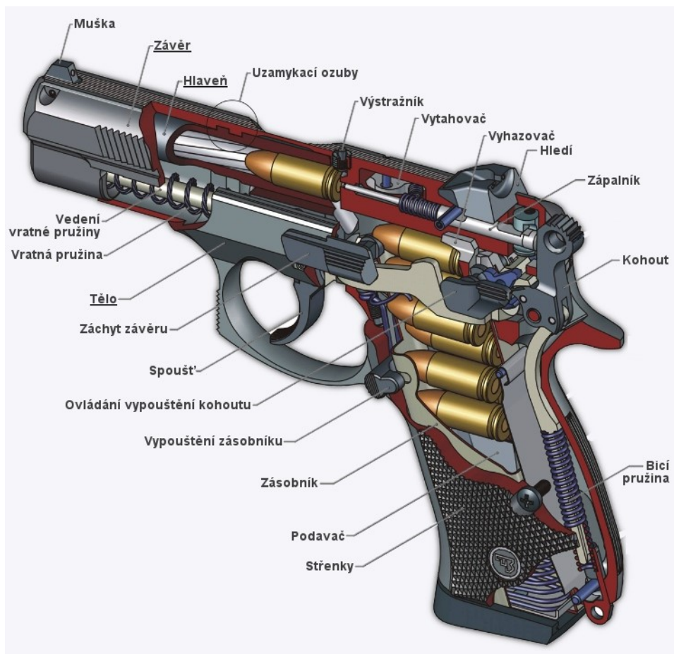
Obr. 1. Krátká kulová zbraň – CZ 75 s popisem komponent [29]
