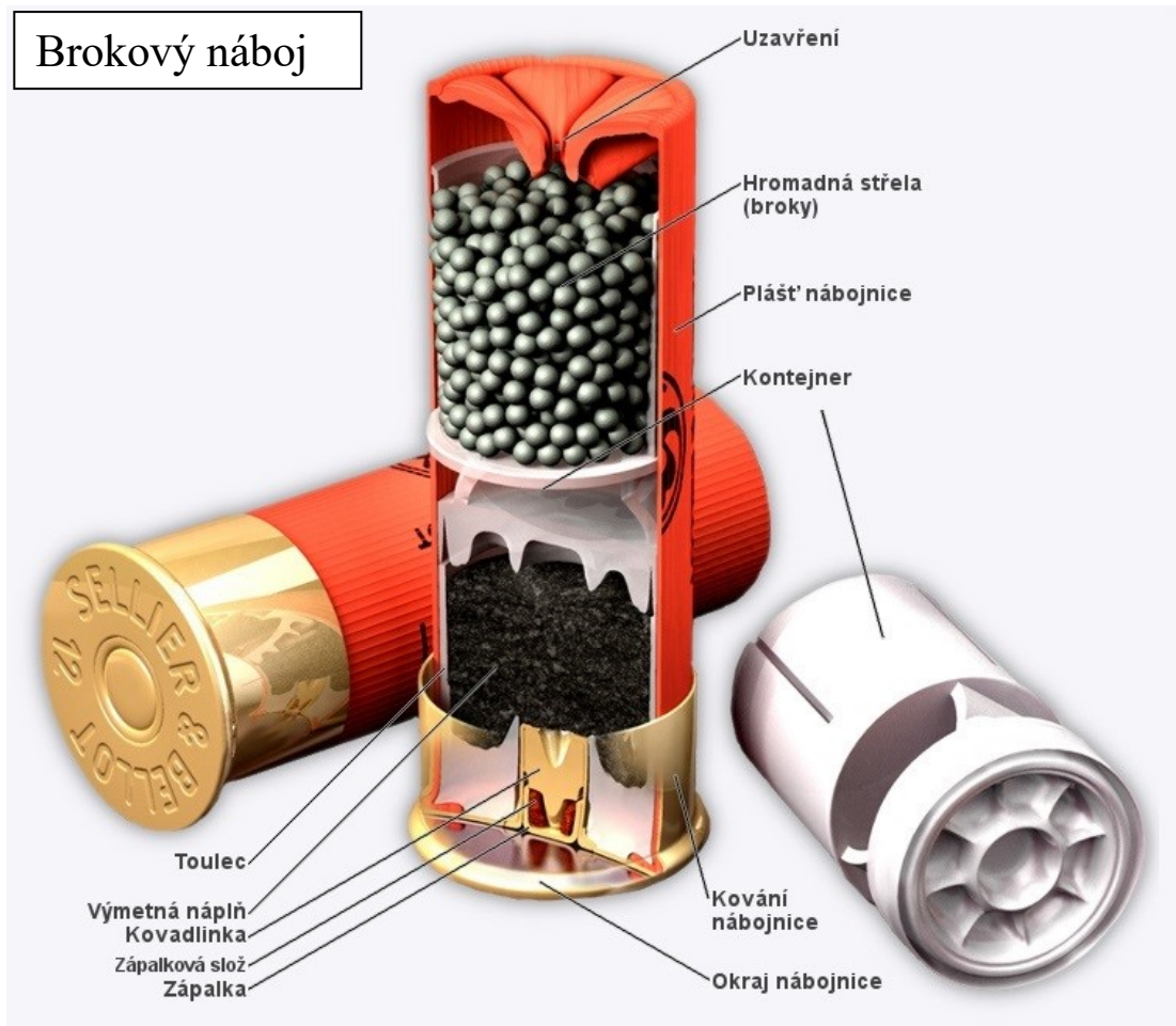
Obr. 3. Brokový náboj s hromadnou střelou a jeho popis [31]
