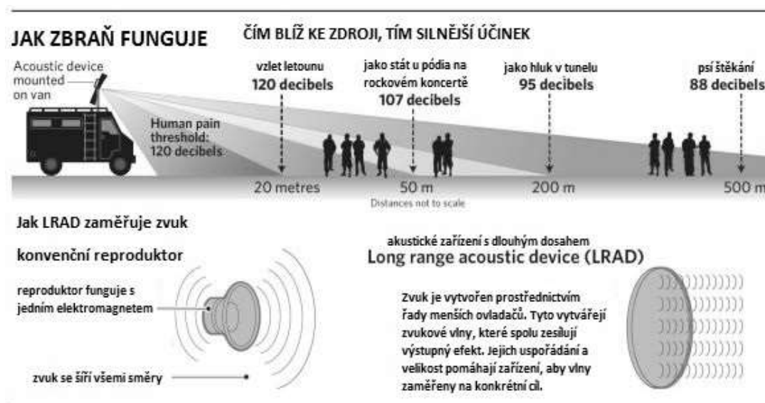
Obrázek 7: vyobrazení fungování zařízení LRAD
